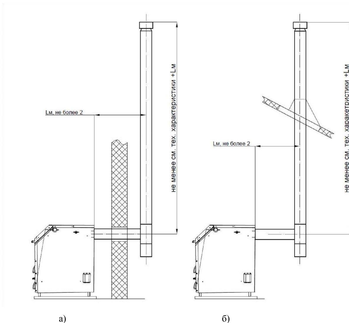
Рисунок 5 - Рекомендуемые схемы дымохода
